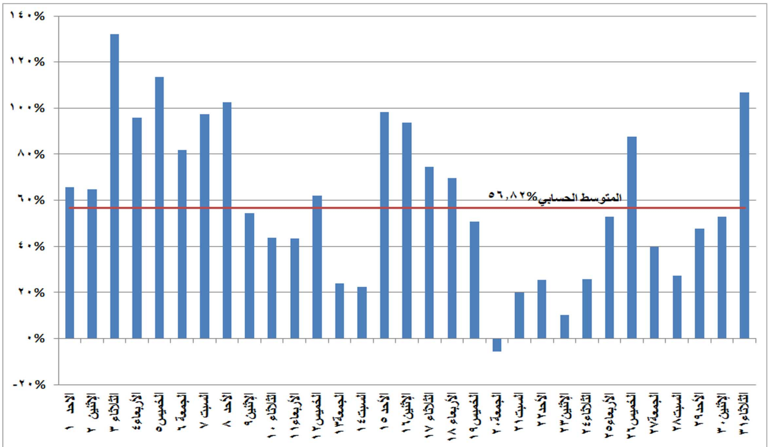
شكل (٢٢) نسب التغير في استخدام المصادر غير الحرارية في إنتاج الطاقة الكهربائية خلال شهر ديسمبر ٢٠١٩ مقارنة بالشهر المماثل من العام السابق
