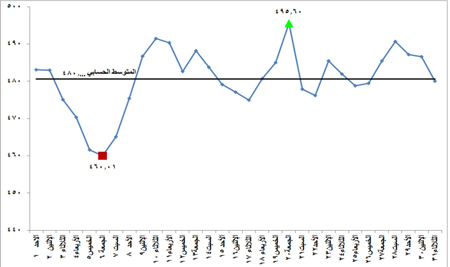
شكل (١٤) معامل انبعاثات غاز ثاني اكسيد الكربون المكافئ على مدى شهر ديسمبر ٢٠١٩
