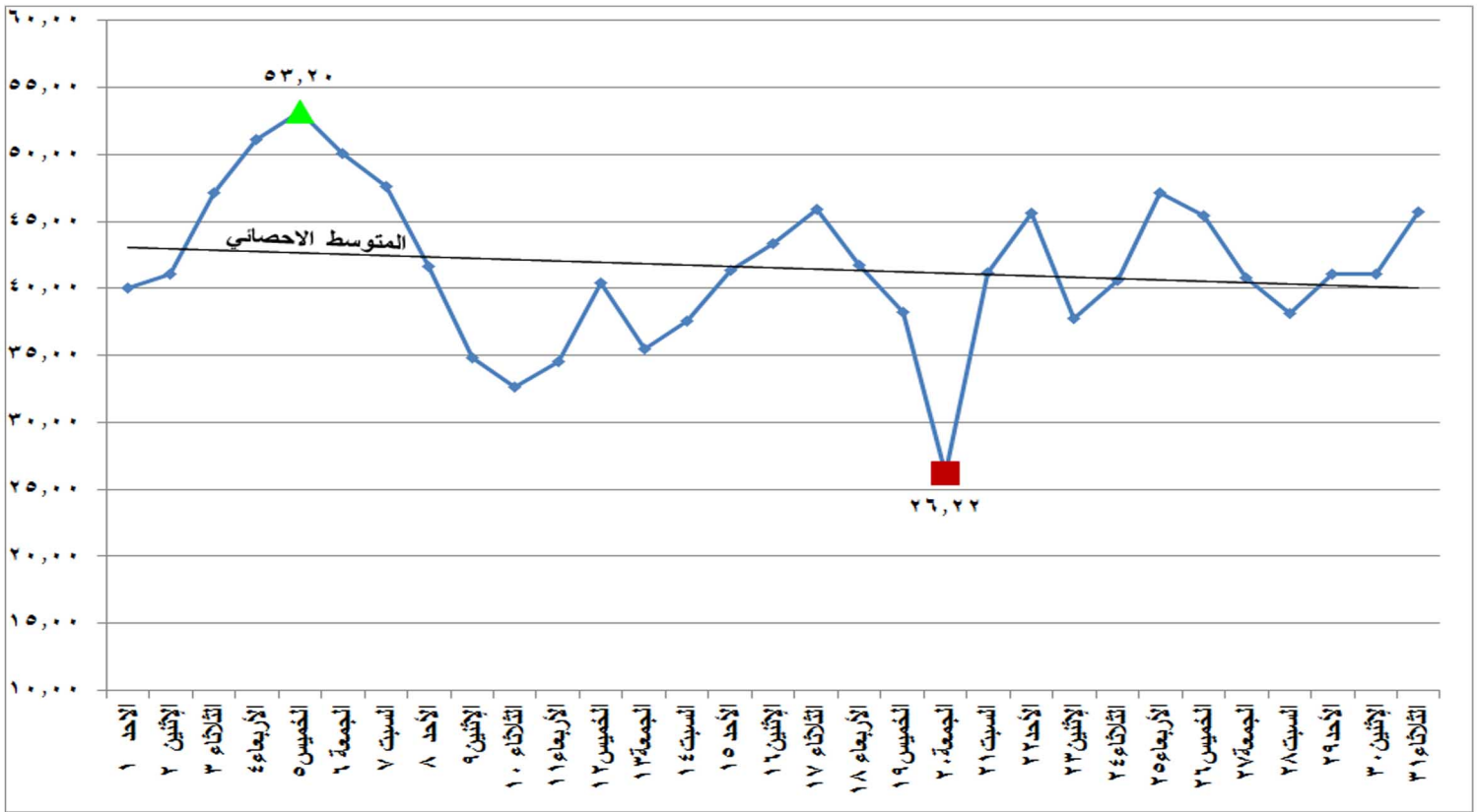
شكل (٢١) الطاقة الكهربائية المنتجة من المصادر غير الحرارية خلال شهر ديسمبر ٢٠١٩
