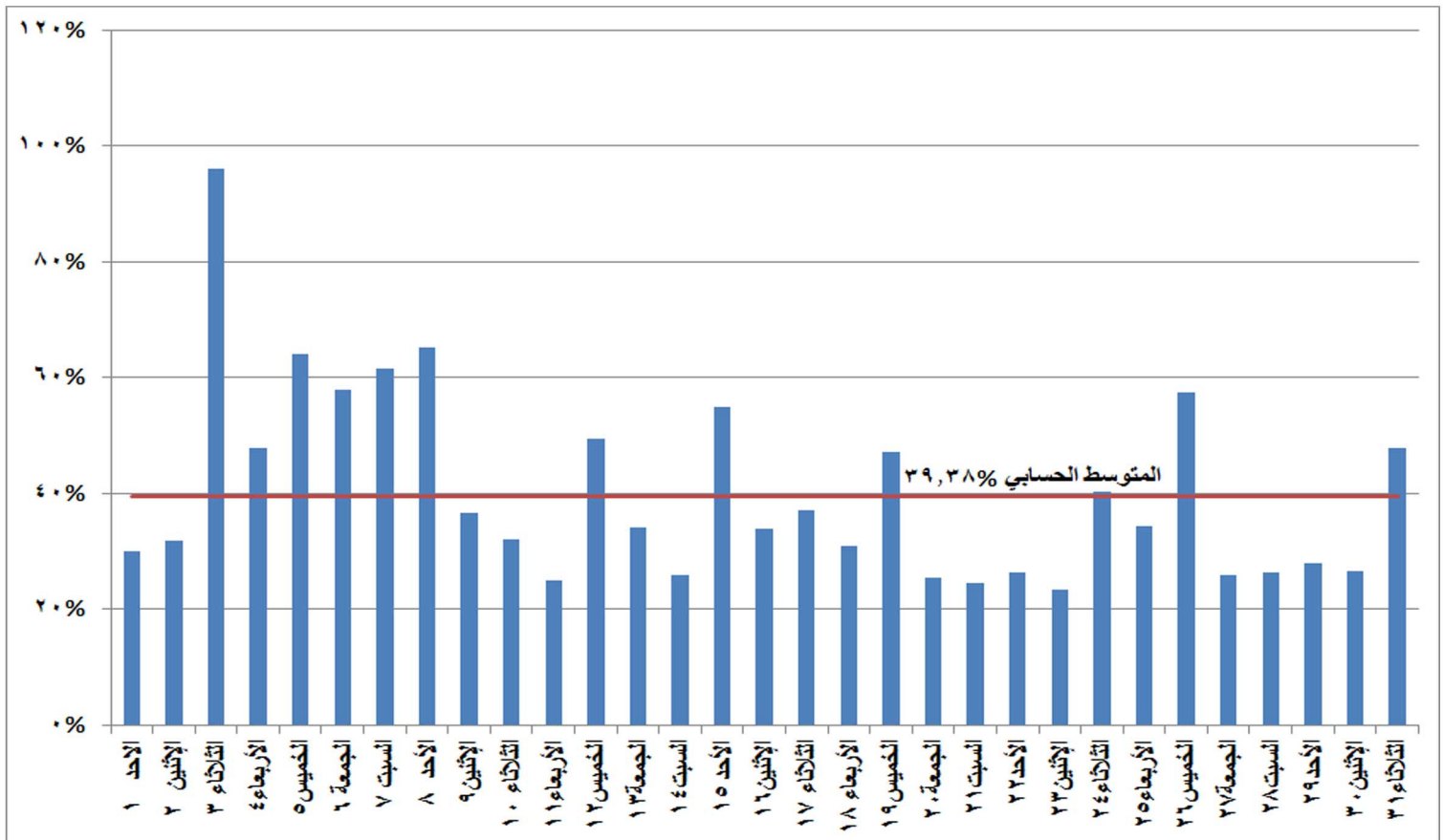
شكل (٢٤) نسب التغير في استخدام المصادر المائية في إنتاج الطاقة الكهربائية خلال شهر ديسمبر ٢٠١٩ مقارنة بالشهر المماثل من العام السابق
