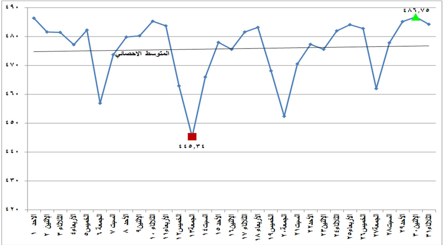
شكل (١٥) إجمالي الطاقة الكهربائية المنتجة من كل المصادر الأولية خلال شهر ديسمبر ٢٠١٩
