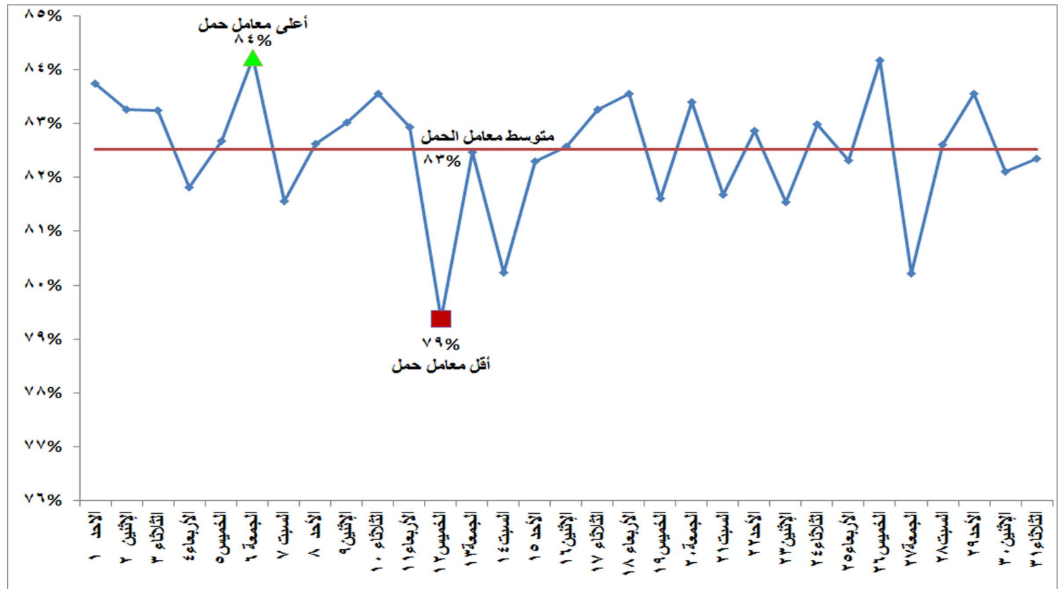
شكل (١٢) إجمالي معامل الحمل لوحدات الانتاج خلال شهر ديسمبر ٢٠١٩
