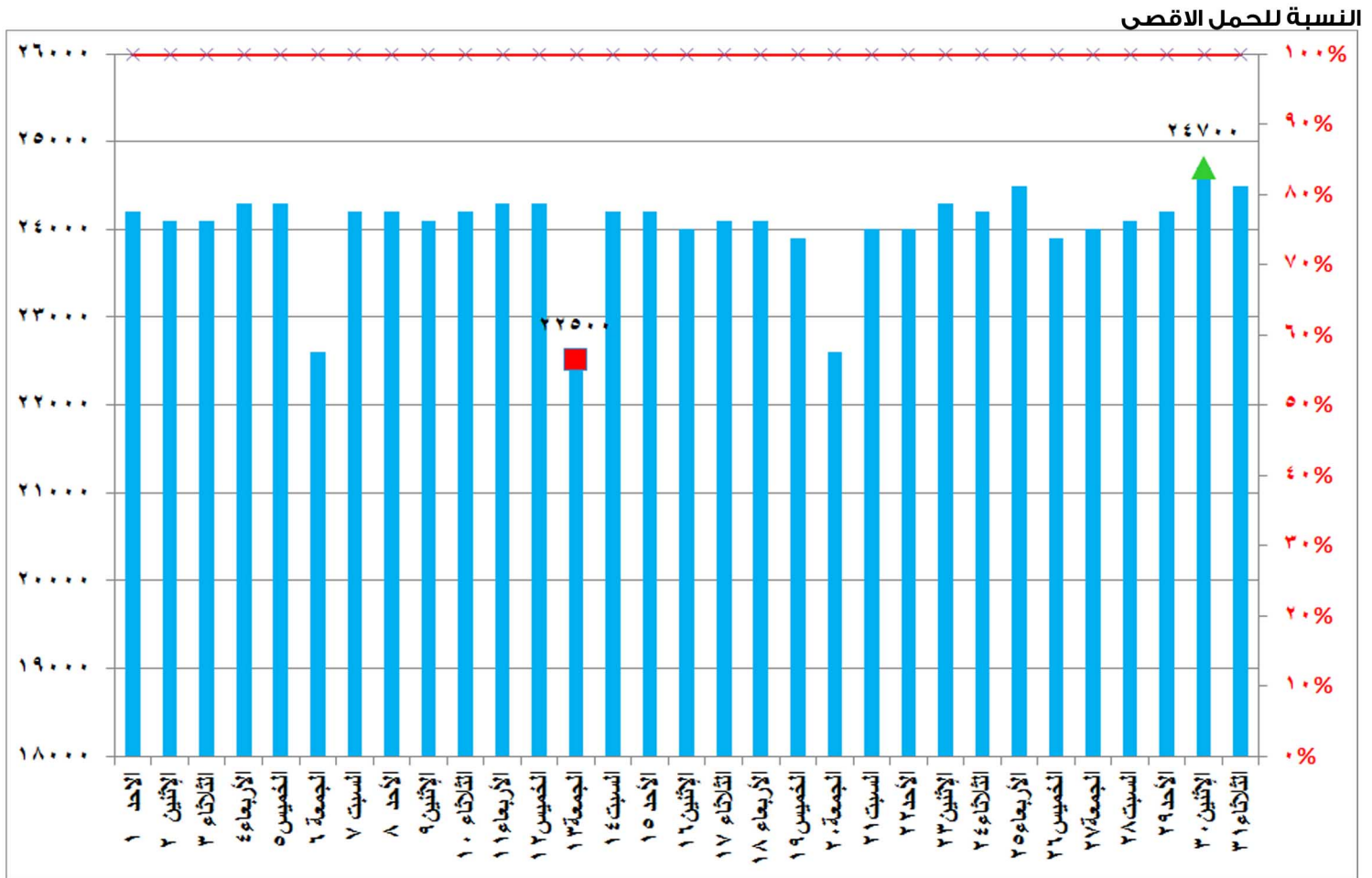
شكل (٥) قدرات الانتاج المتاحة ونسبتها للحمل الأقصى خلال شهر ديسمبر ٢٠١٩
