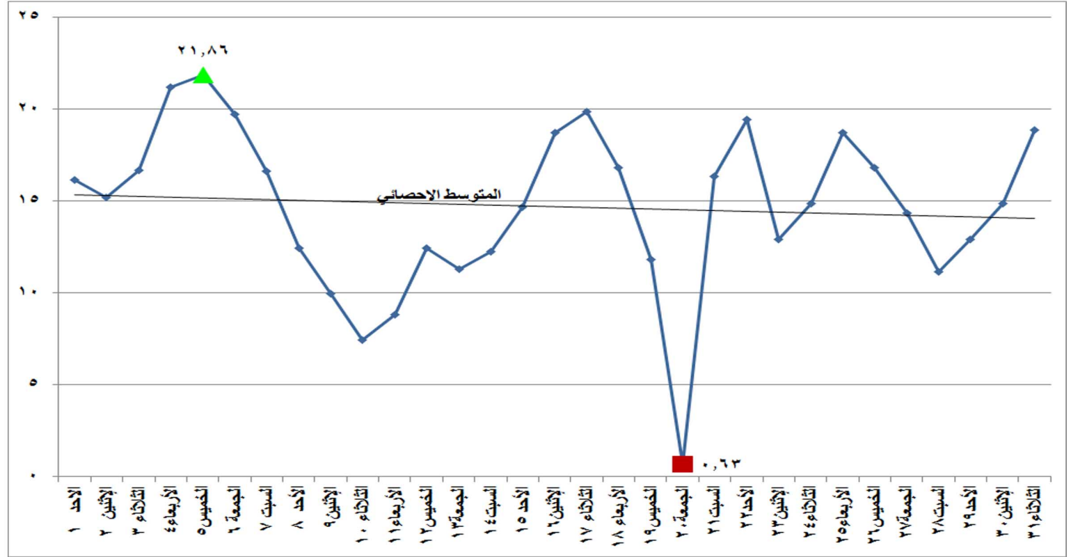
شكل (٢٥) الطاقة الكهربائية المنتجة من الرياح والشمس خلال شهر ديسمبر ٢٠١٩
