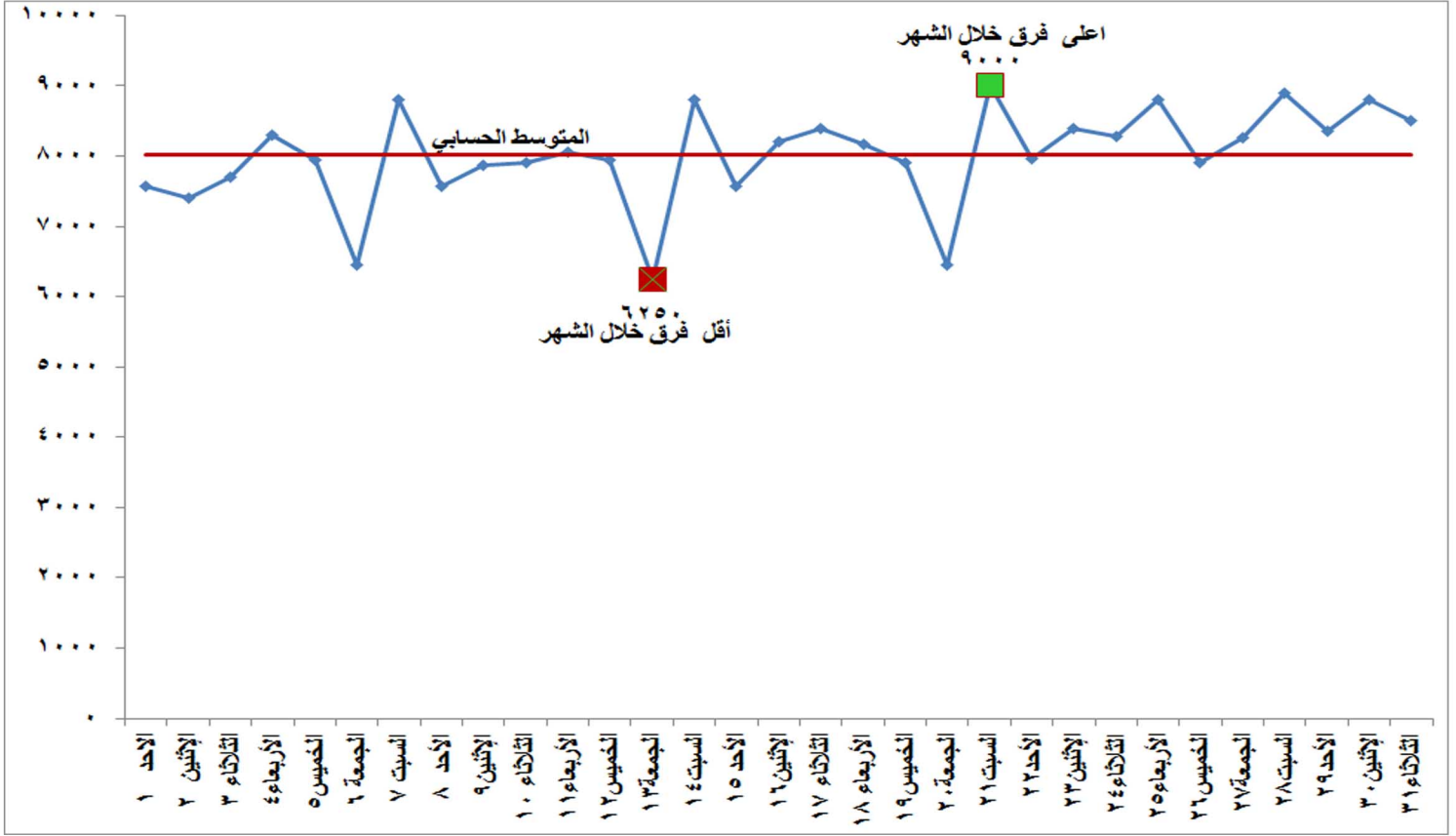
شكل (٣) الفرق بين أقصى وأدنى حمل خلال شهر ديسمبر ٢٠١٩
