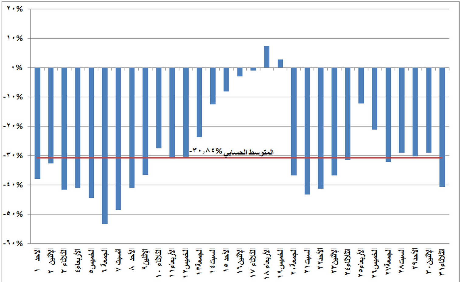
شكل (٢٠) نسب التغير في استخدام المازوت في إنتاج الطاقة الكهربائية خلال شهر ديسمبر ٢٠١٩ مقارنة بالشهر المماثل من العام السابق
