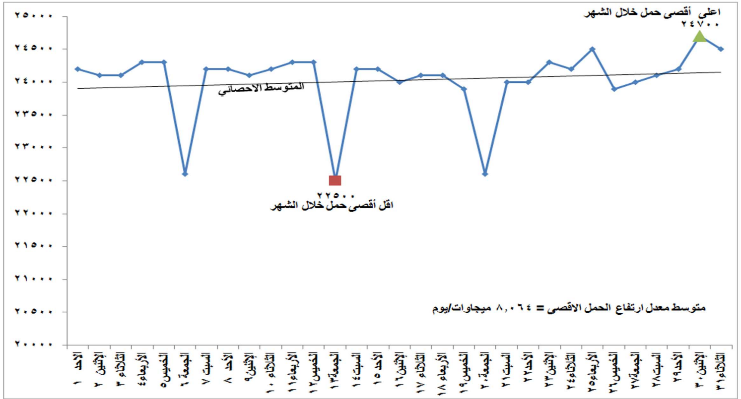
شكل (١) تطور الحمل الاقصى اليومي خلال شهر ديسمبر ٢٠١٩
