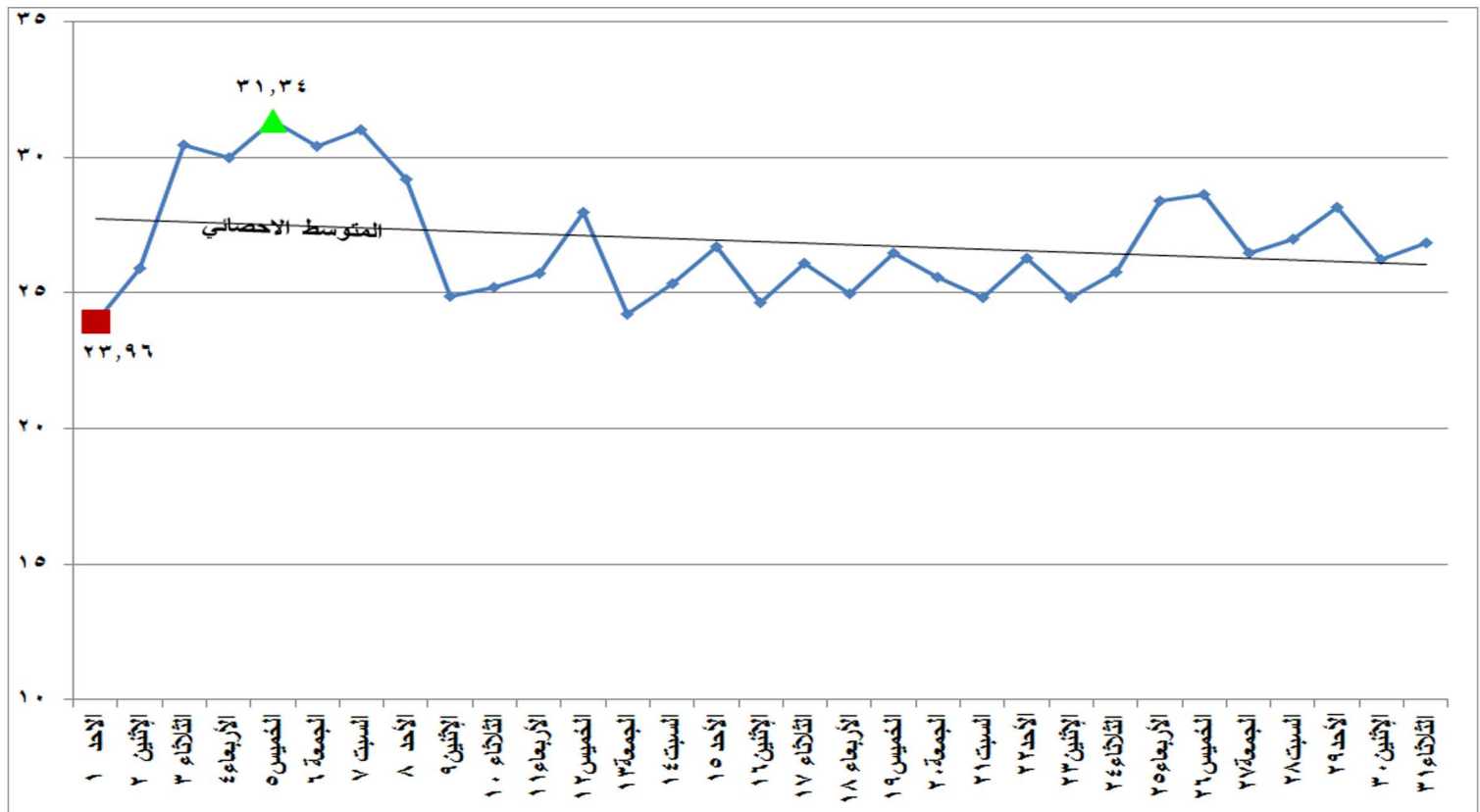
شكل (٢٣) الطاقة الكهربائية المنتجة من المصادر المائية خلال شهر ديسمبر ٢٠١٩
