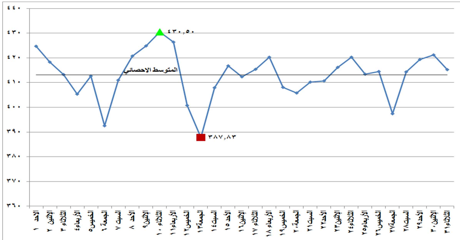
شكل (١٧) الطاقة الكهربائية المنتجة من الغاز الطبيعي خلال شهر ديسمبر ٢٠١٩
