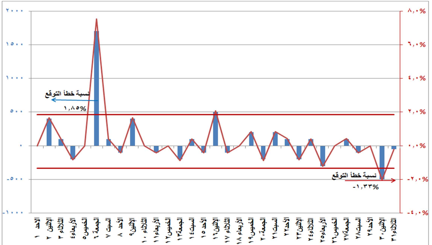
شكل (١٠) الفرق بين الحمل الأقصى المتوقع والمسجل فعليا ونسبة الفرق إلى الحمل المسجل فعليا خلال شهر ديسمبر ٢٠١٩
