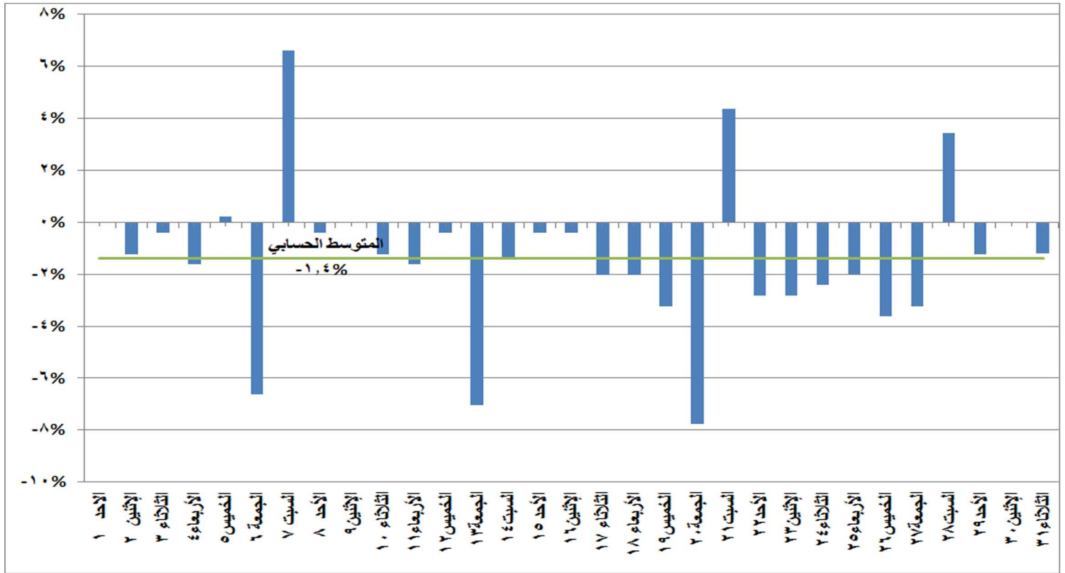
شكل (٩) النسب المئوية للتغير في الحمل الاقصى خلال شهر ديسمبر ٢٠١٩ مقارنة باليوم المماثل من العام الماضي
