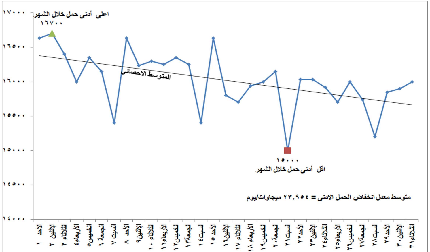
شكل (٢) تطور الحمل الادنى اليومي خلال شهر ديسمبر ٢٠١٩
