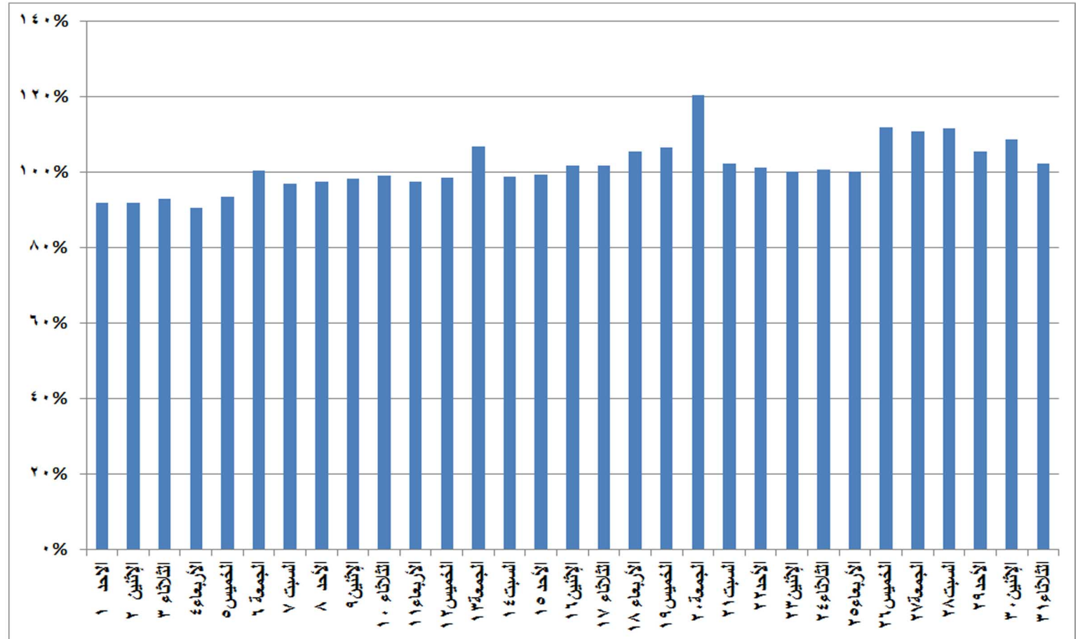
شكل (٢٨) نسب الفائض للحمل الاقصى المسجل يوميا خلال شهر ديسمبر ٢٠١٩
